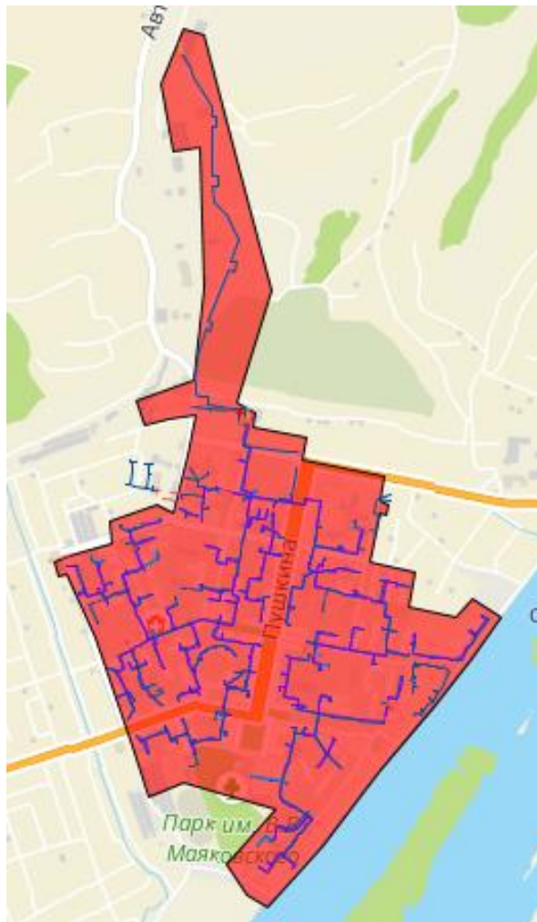
Рисунок 1.7 – Зона действия Абашевской районной котельной
