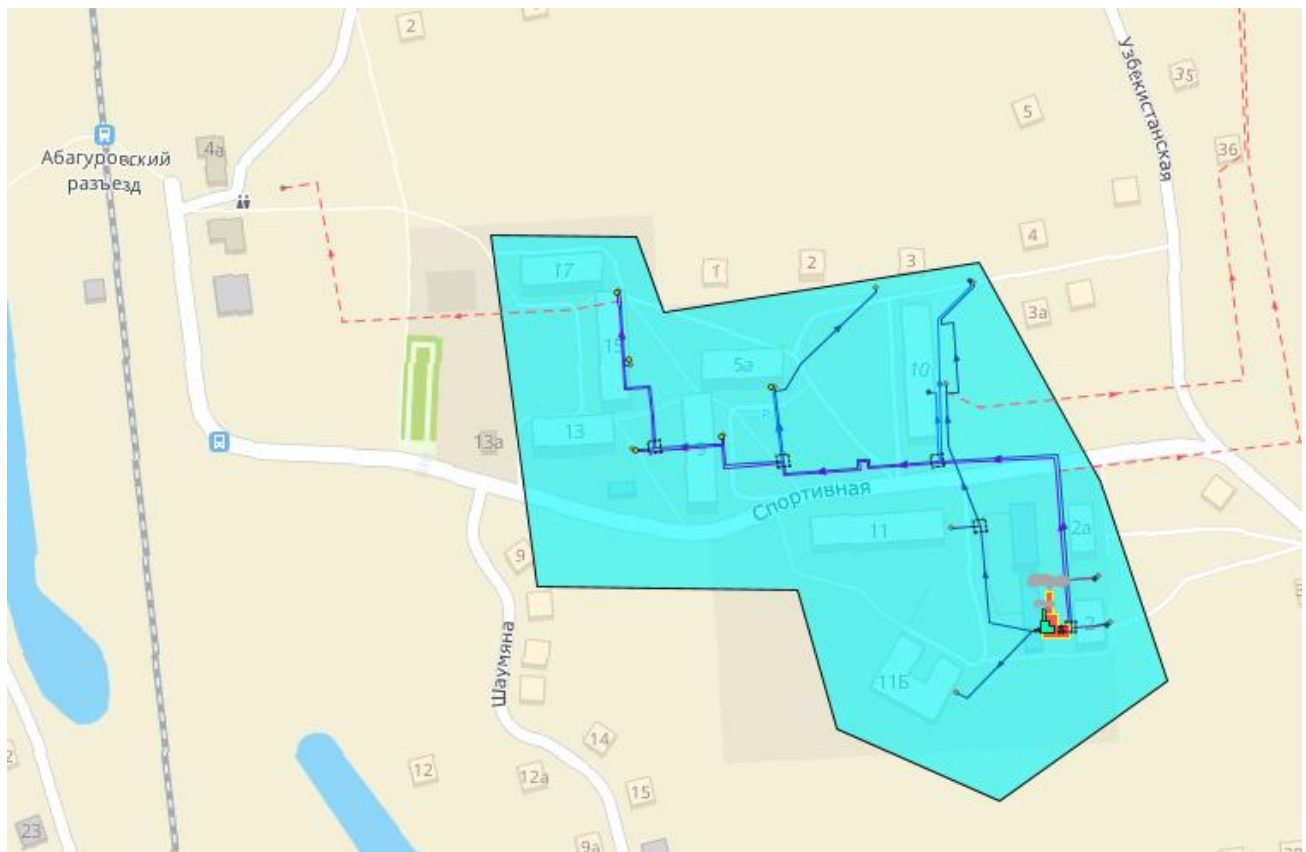
Рисунок 1.23 – Зона действия котельной №2 п. Разъезд-Абагуровский
