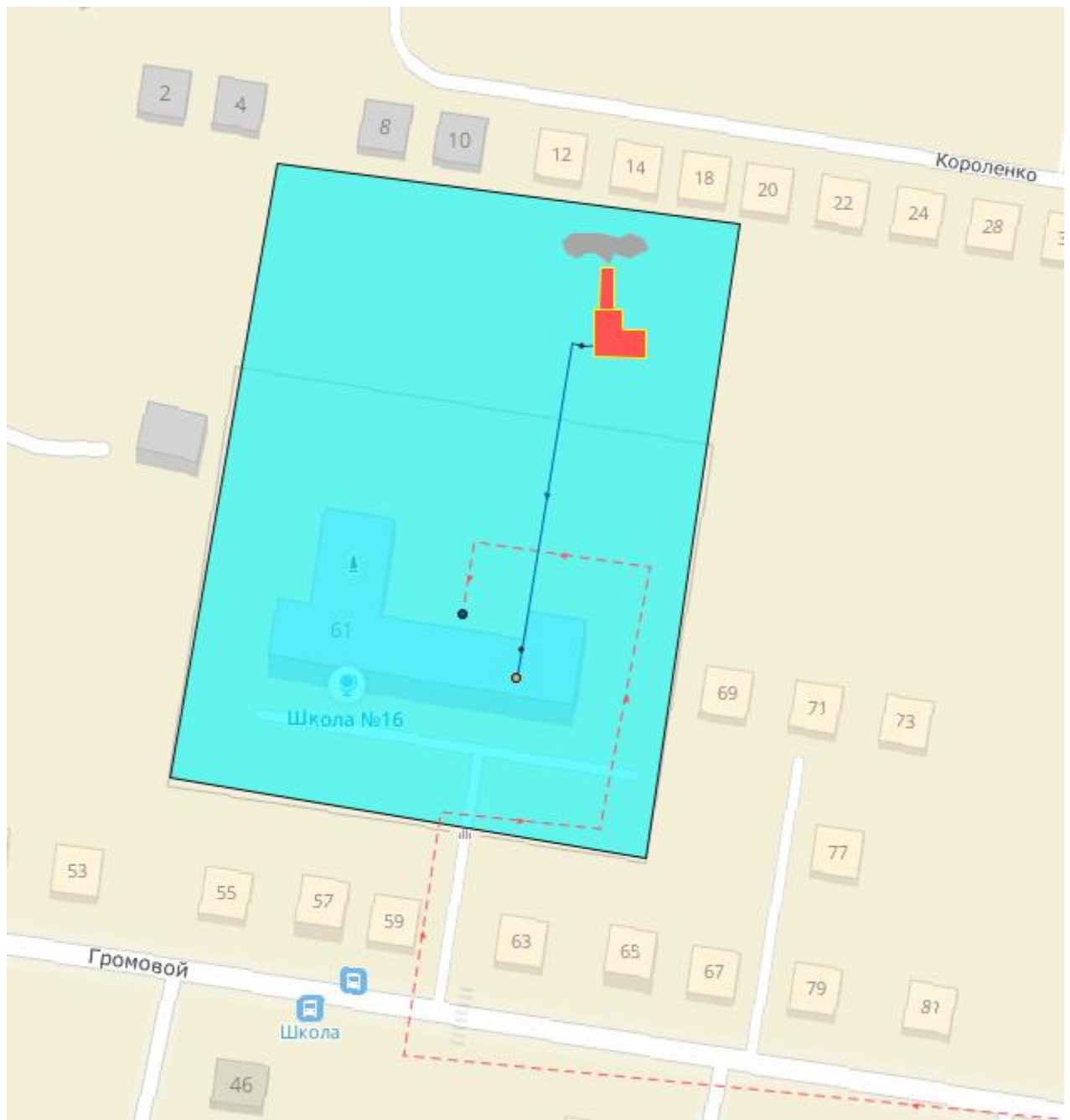
Рисунок 1.32 – Зона действия котельной Школы №16
