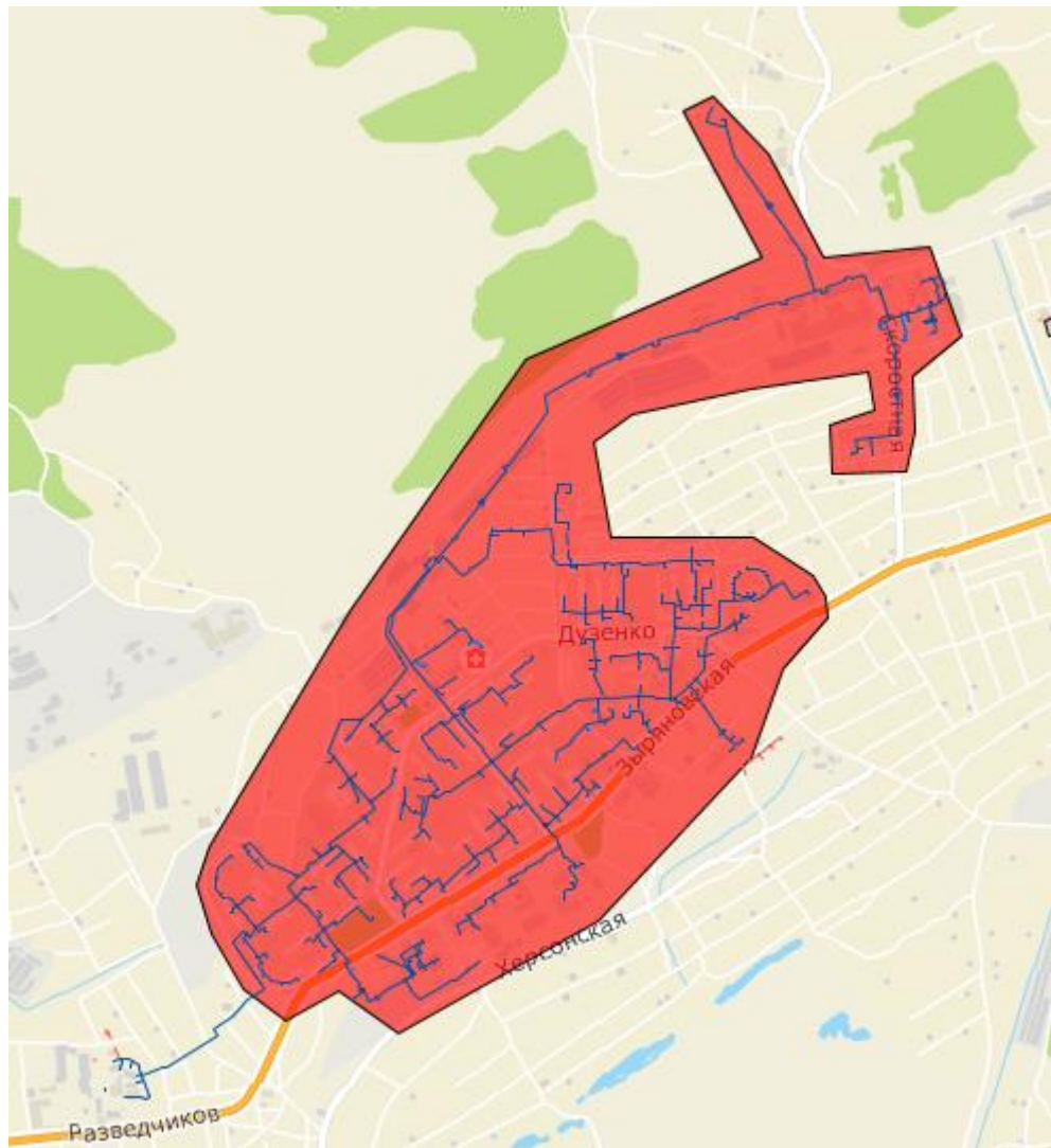
Рисунок 1.9 – Зона действия Зыряновской районной котельной
