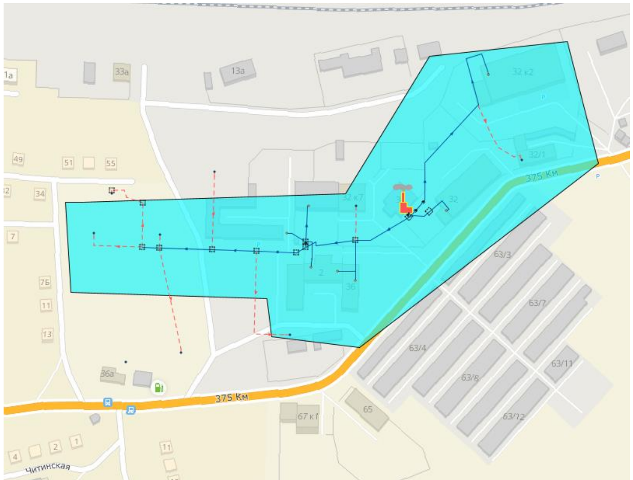
Рисунок 1.20 – Зона действия котельной №6
