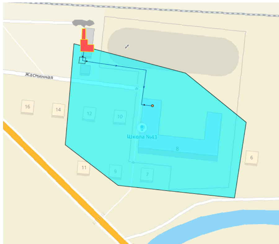
Рисунок 1.30 – Зона действия котельной школы №43
