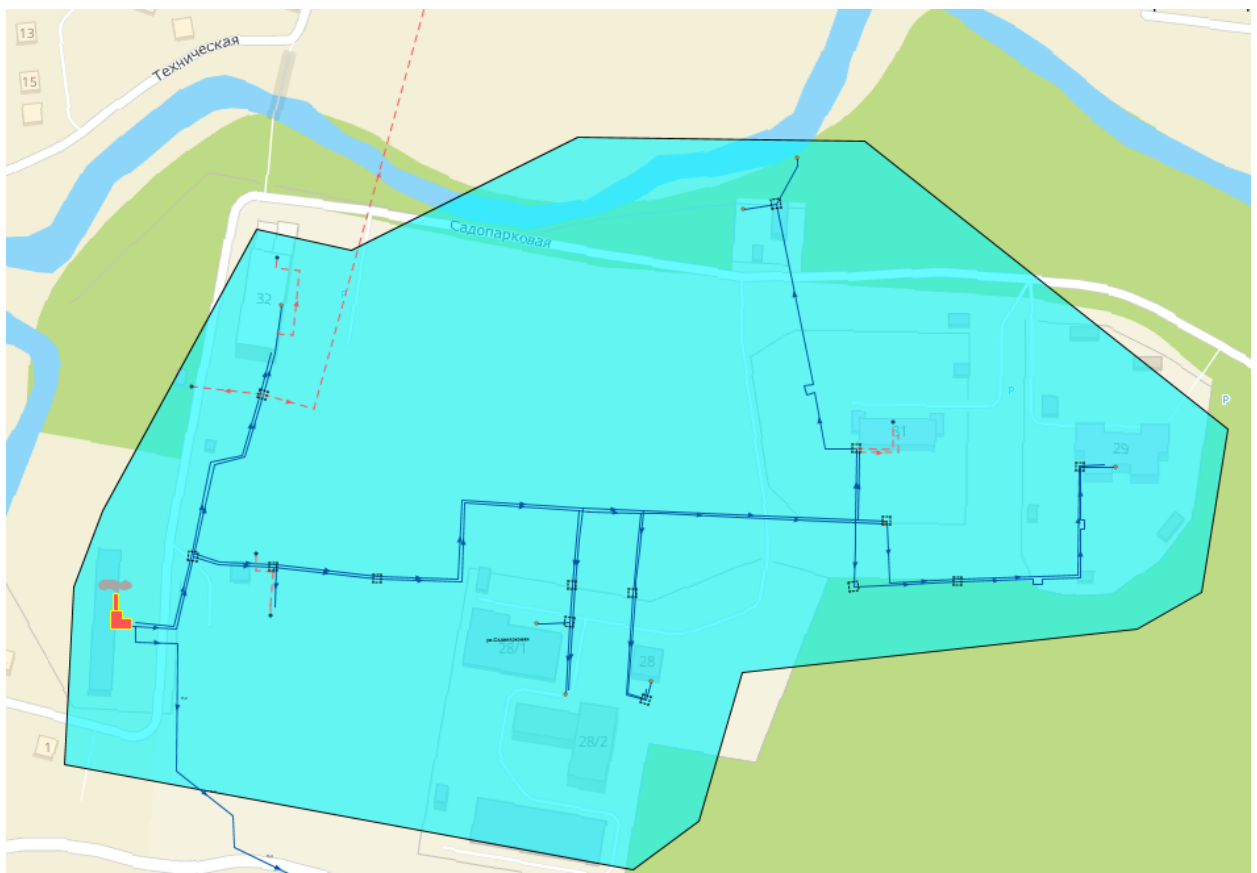
Рисунок 1.21 – Зона действия котельной №32 (БПОУ)
