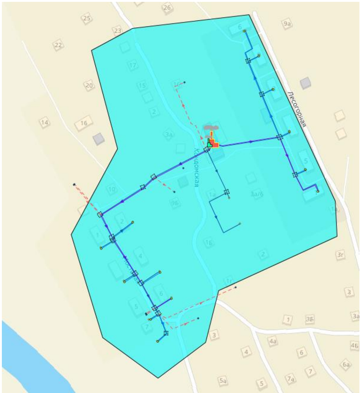
Рисунок 1.22 – Зона действия котельной №1 п. Разъезд-Абагуровский
