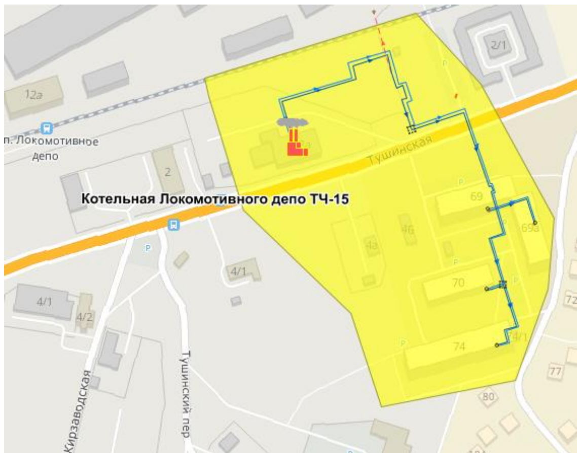
Рисунок 1.38 – Зона действия котельной Локомотивного депо ТЧ-15 ст. Новокузнецк-Сортировочный (ДВТУ-3)
