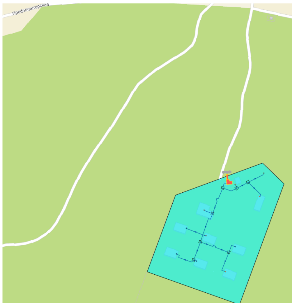
Рисунок 1.31 – Зона действия котельной интерната №66 (Монтажник)
