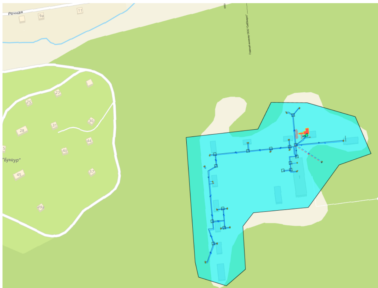
Рисунок 1.24 – Зона действия котельной проф. «Бунгурский»
