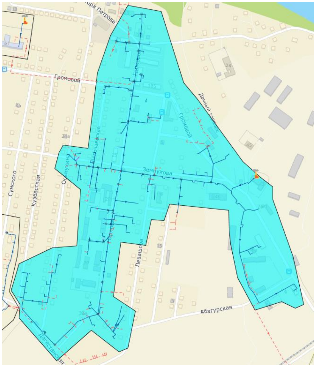
Рисунок 1.16 – Зона действия котельной №1 п. Абагур-Лесной
