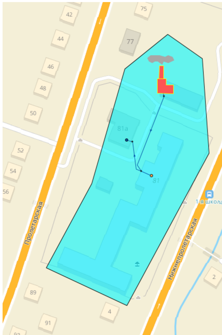
Рисунок 1.27 – Зона действия котельной школы №1
