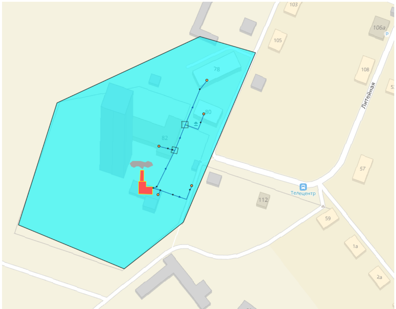
Рисунок 1.25 – Зона действия котельной «РТРС»
