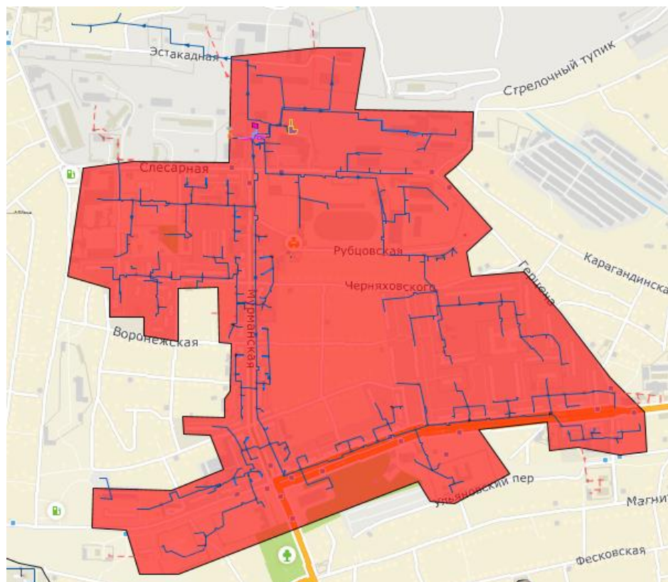
Рисунок 1.8 – Зона действия Байдаевской центральной котельной №2
