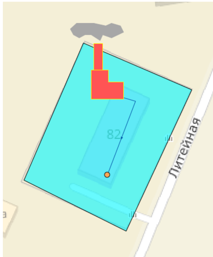
Рисунок 1.33 – Зона действия котельной детского сада №123
